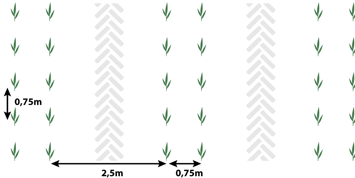
Plantafstand biomassateelt populier. Teeltsysteem met dubbele plantrijen en een 3-jarige oogstcyclus (8.500 stekken per hectare)
