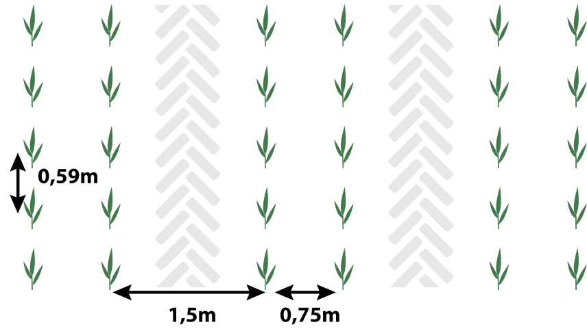
Plantafstand biomassateelt wilg. Teeltsysteem met dubbele planrijen en een 1 tot 4-jarige oogstcyclus (15.000 stekken per hectare)
