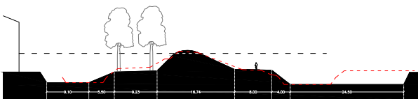
Bestaande situatie A-A'
