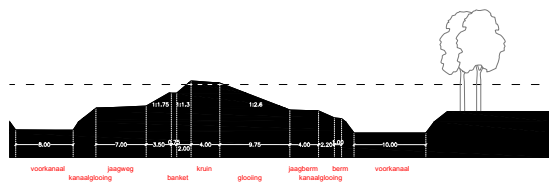
oorspronkelijk profiel Geniedijk
