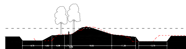
Bestaande situatie B-B'
