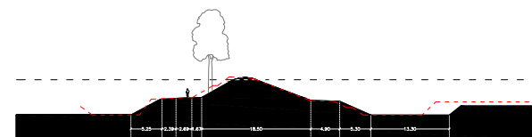
Bestaande situatie C-C'
